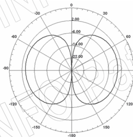
E-Plane
