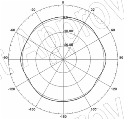
H-Plane
