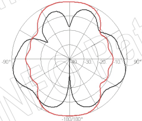
H-Plane
