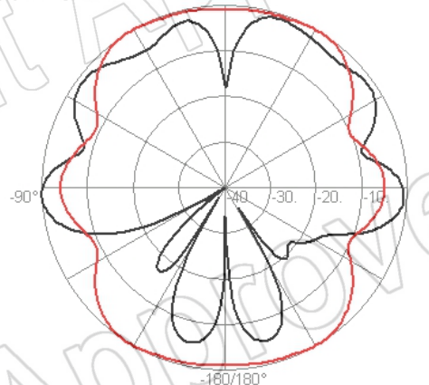
H-Plane
